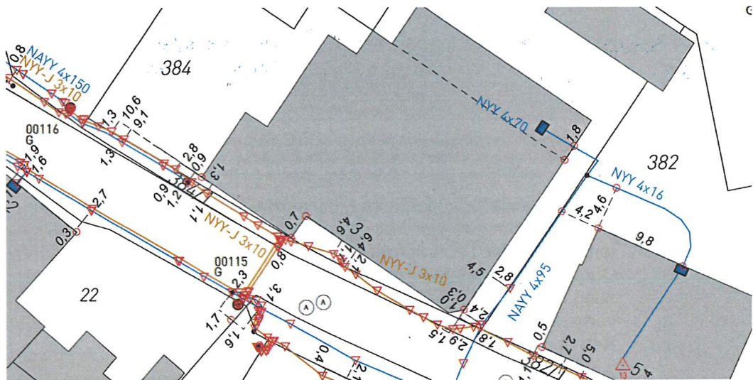
Leitungsplan der Netze BW GmbH aus der Stellungnahme vom 27.07.2020
